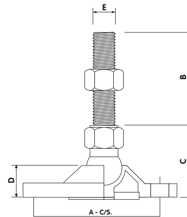
BOLT DOWN A-JUSTA-FOOT
